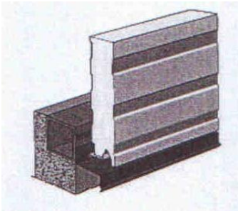
детал на фасаден панел (детал укрутување долу)
