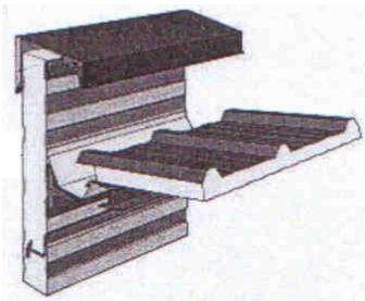
детал за изведба на атика
